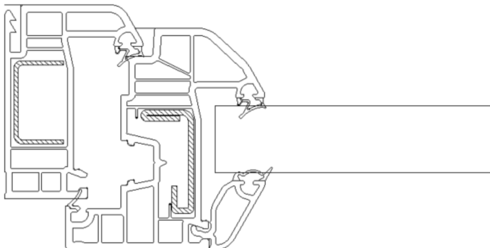
Figure 4 : Dormant 711-28 – Ouvrant 722-13
