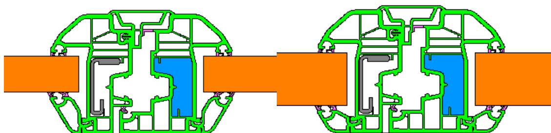
Figure 11 : Ouvrants 722-13M – 722-14 + Battement 741-40
