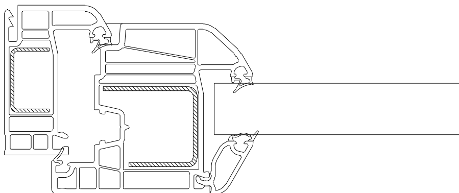
Figure 8 : Dormant 711-28 – Ouvrant 722-15
