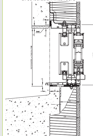
Possibilité de dormant monobloc 100/120/140/160 mm
